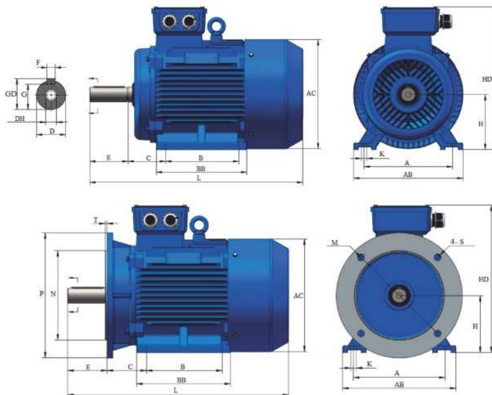
Габаритные, установочные и присоединительные размеры двигателей.
